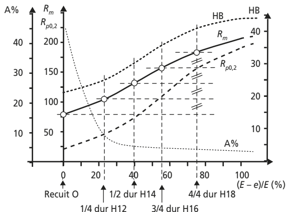
Figure 10.10 Évolution schématique des propriétés mécaniques de l'aluminium 1050 avec son taux d'écrouissage.
