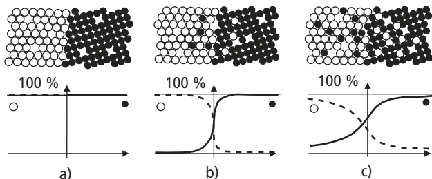
Figure 3.21 Interdiffusion progressive de deux solides purs et profils de concentration correspondants.
