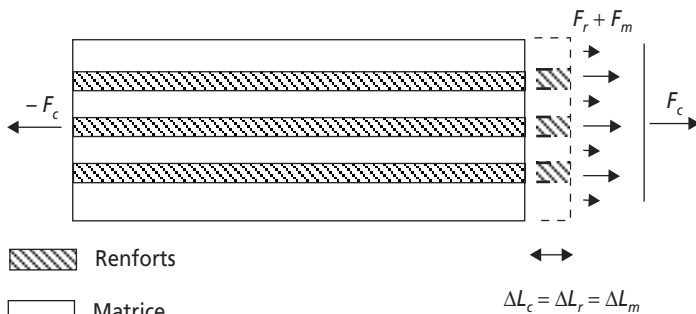
Figure 13.1 Barreau en composite à fibres longues sollicité dans la direction longitudinale.
