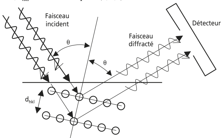
Figure 3.30 Diffraction d'une onde incidente par une famille de plans atomiques d'un cristal.
