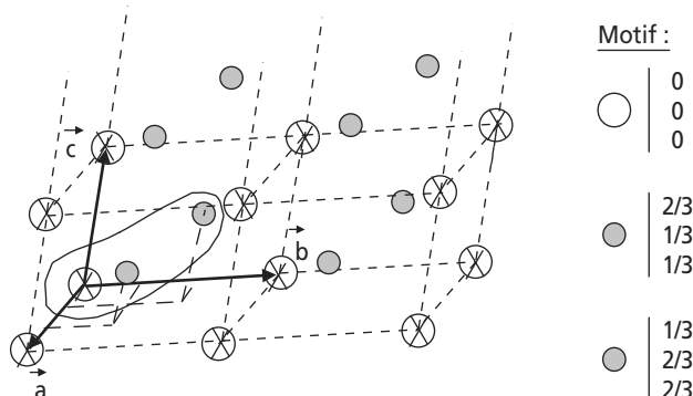
Figure 3.6 Exemple de motif atomique comportant trois atomes.
