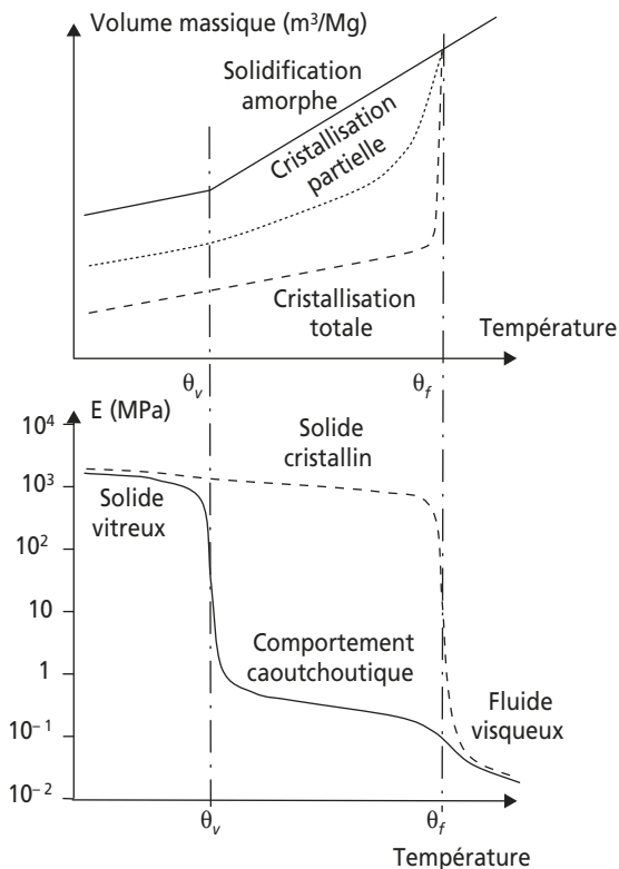
Figure 11.4 Évolutions schématisques du volume massique V_m et du module de Young E d'un polymère en fonction de la température.
