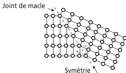
Figure 3.17 Schématisation à deux dimensions d'un joint de macle.
