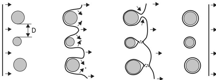
Figure 6.11 Mécanisme d'Orowan :
