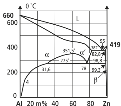
Figure 4.9 Exemples de diagrammes de phases binaires. (Suite)
