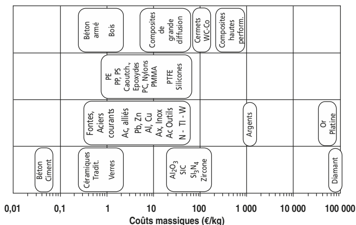
Figure 14.3 Ordres de grandeur des coûts massiques des principaux matériaux avant mise en œuvre.
