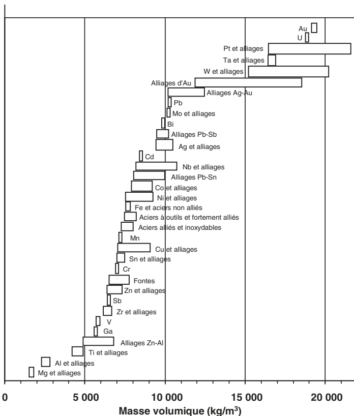
Figure 10.17 Masse volumique des principales familles d'alliages métalliques.
