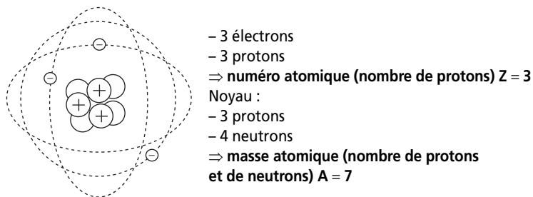
Figure 2.1 Exemple de l'atome de lithium.
