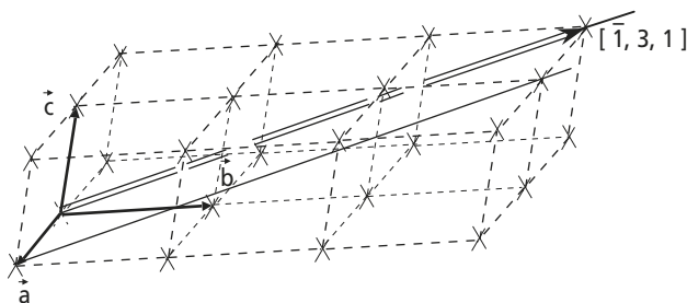
Figure 3.7 Exemple d'indice de direction cristallographique : la direction [1, 3, 1] est celle de la rangée atomique qui joint le nœud origine au nœud de coordonnées -1, +3, +1 (le signe « - » est inscrit au-dessus de l'indice négatif par souci de gain de place dans la notation).
