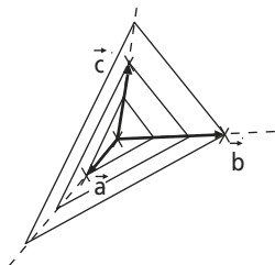
Figure 3.8 Exemple de plan cristallographique, famille de plans parallèles équidistants. Les plans tracés découpent un segment sur le vecteur \vec{a} , trois segments égaux sur le vecteur \vec{b} , deux segments égaux sur le vecteur \vec{c} : les indices de ce plan cristallographique sont (1, 3, 2).
