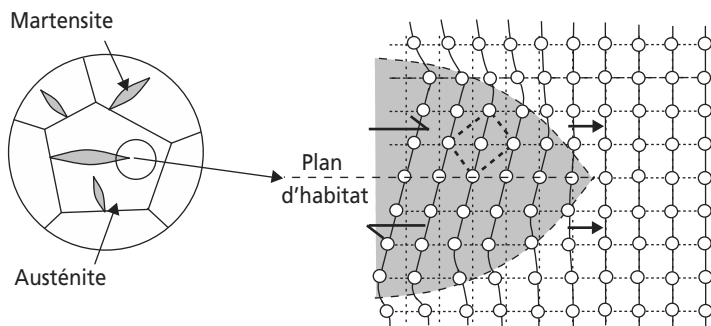
Figure 5.8 Représentation schématisée simplifiée du mécanisme de la transformation martensitique du fer.
