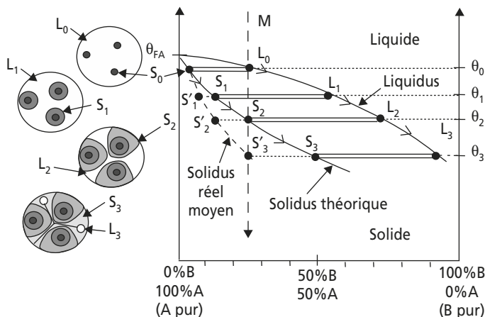
Figure 5.6 Apparition de ségrégations mineures et abaissement de la température de solidification au cours d'une solidification non isotherme.
