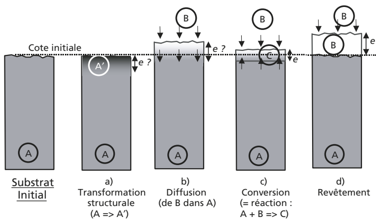
Figure 13.8 Les quatre types de traitements de surface.
