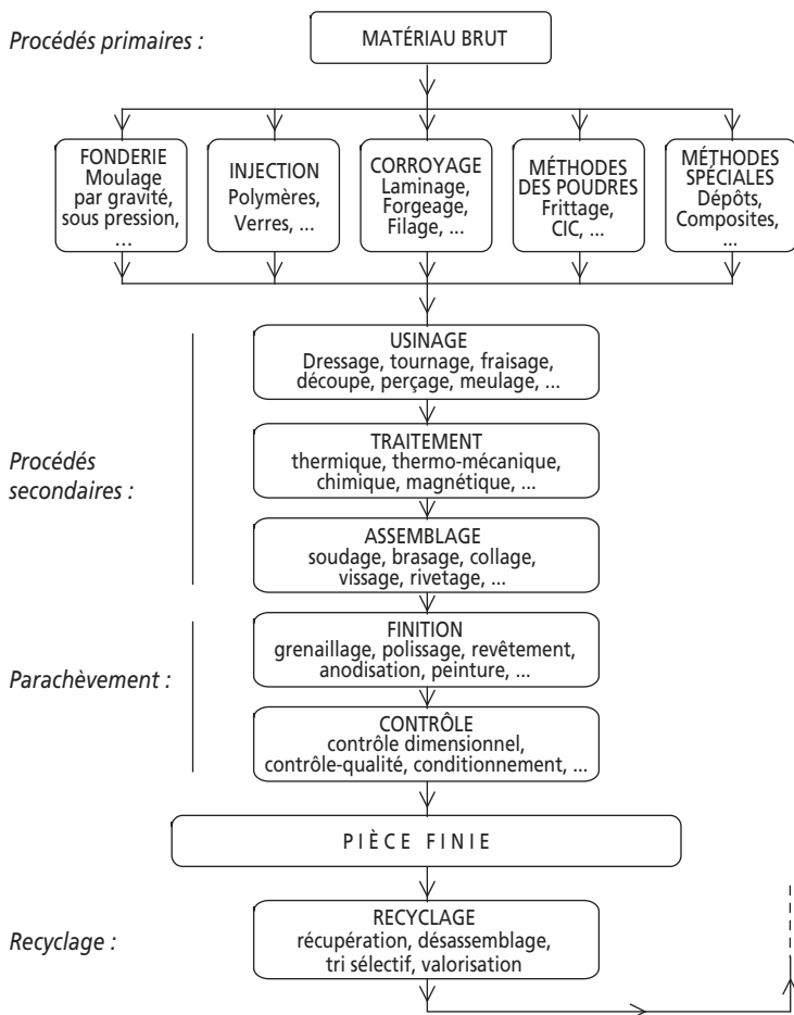
Figure 14.4 Classification schématique des procédés selon leur méthodologie de mise en œuvre.
