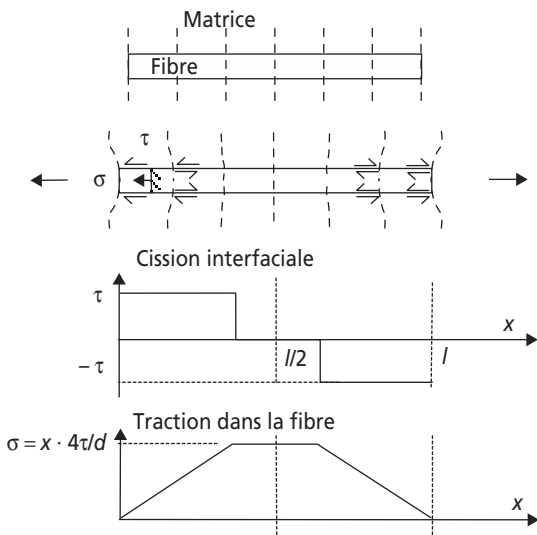
Figure 13.2 Transfert de charge depuis la matrice vers une fibre courte par les cisssions interfaciales.
