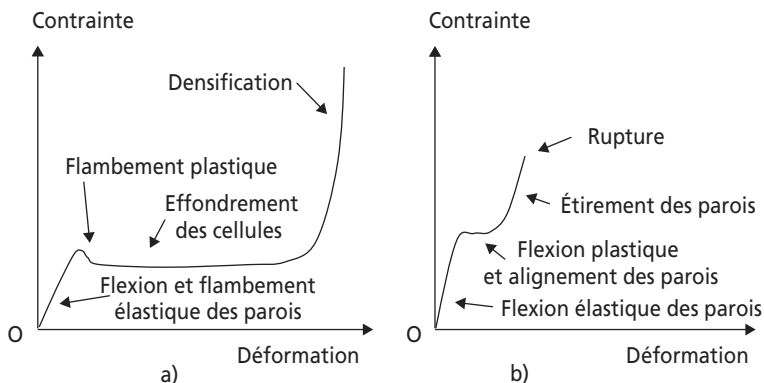
Figure 13.9 Comportement mécanique d'une mousse : a) en compression; b) en traction.
