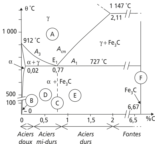
Figure 10.4 Diagramme de phases des aciers au carbone non alliés (voir tableau 10.13 pour les microstructures).
