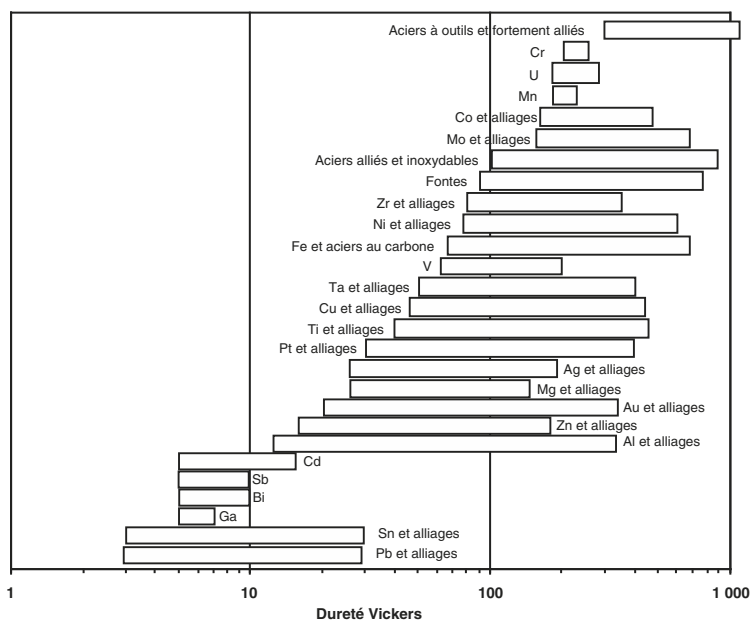
Figure 10.18 Dureté Vickers des principales familles d'alliages métalliques.
