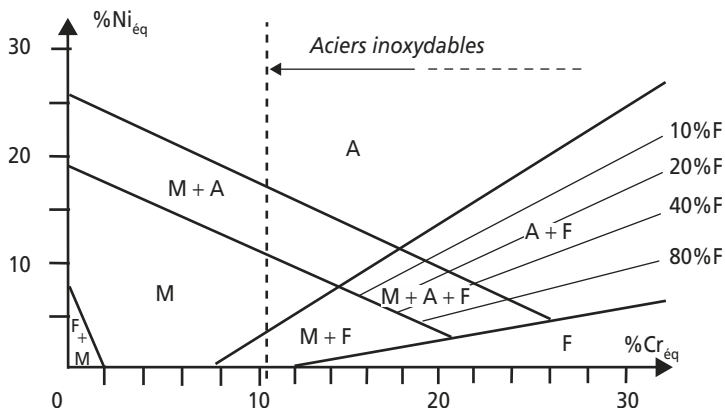
Figure 10.8 Diagramme de Schaeffler, indiquant les phases présentes dans les aciers inoxydables bruts de solidification (ou dans les cordons de soudure) en fonction des pourcentages équivalents en chrome et en nickel.
