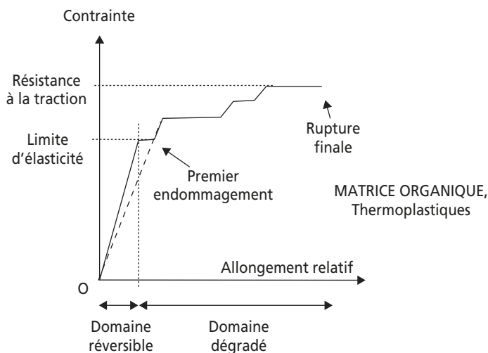
Figure 13.5 Allure de la courbe de traction d'un matériau composite.
