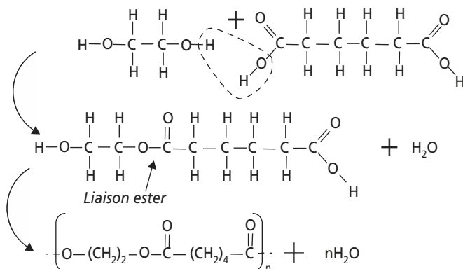
Figure 11.3 Exemple de polycondensation : la polymérisation du polyester à partir de monomères d'éthylène glycol \text{C}_2\text{H}_4(\text{OH})_2 et d'acide adipique \text{C}_6\text{H}_8(\text{OOH})_2 avec formation d'eau.
