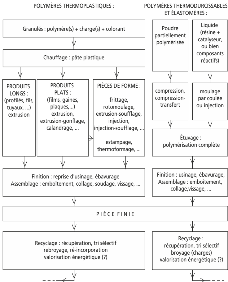
Figure 11.9 Principaux procédés de transformation des polymères thermoplastiques, thermodurcissables et élastomères.
