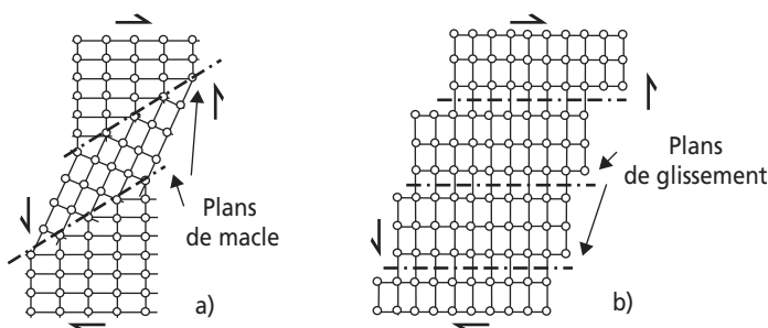
Figure 6.3 Schémas de la déformation d'un cristal : a) par maclage mécanique; b) par glissement.
