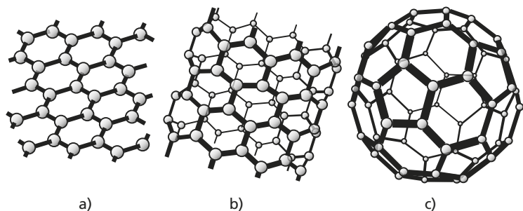
Figure 13.10 Représentation schématique d'un plan de graphène (a), d'un nano-tube de carbone monofeuillet (b) et d'un fullerène C_{60} (c).
