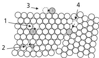
Figure 3.20 Mécanismes de diffusion les plus fréquents dans un solide cristallin.
