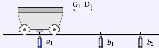
Figure 2.8: Système chariot
